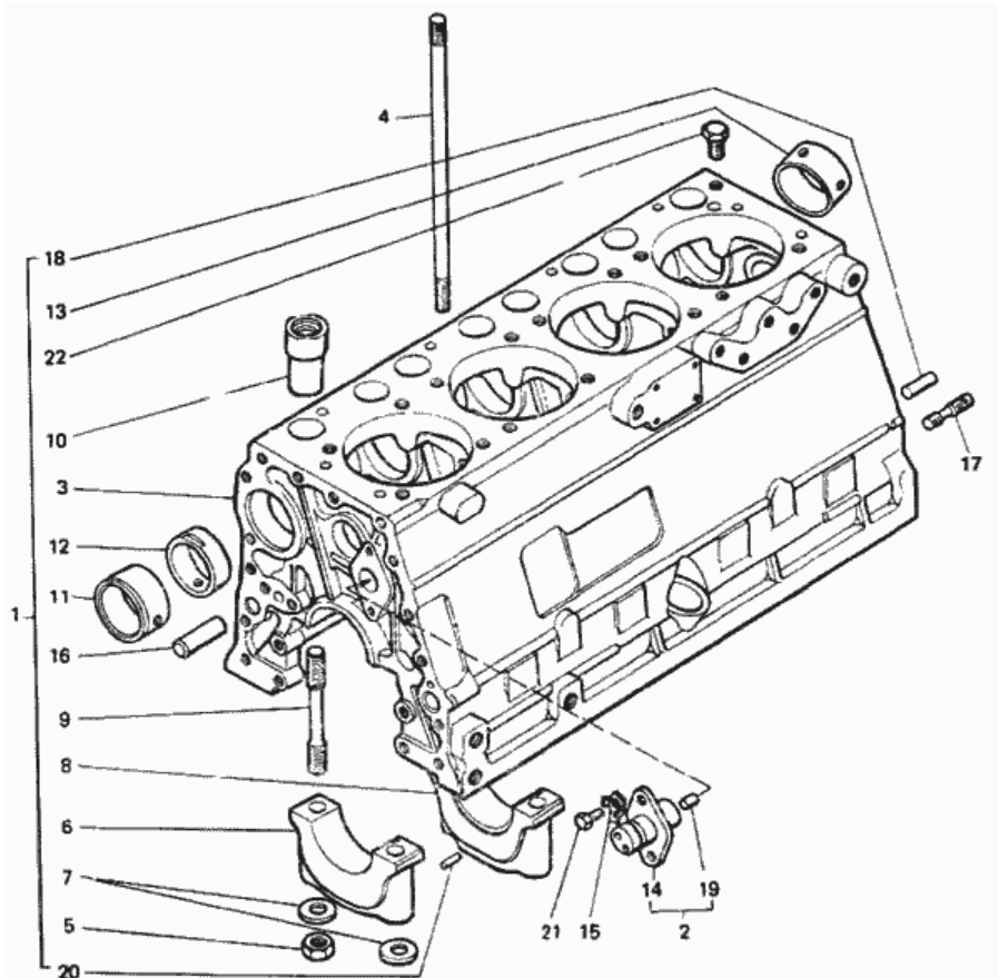
Рис. 16. Картер дизеля Д37М-1002008-А
